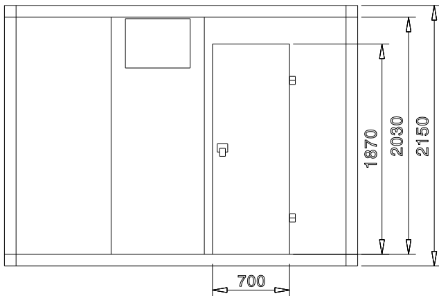
Front aanzicht
